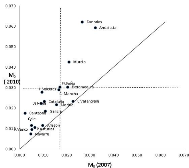
Gráfico 2. Diagrama de dispersión de las comunidades autónomas en relación con sus tasas de pobreza ajustada en 2007 y 2010
