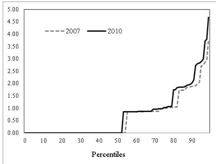
Gráfico 1. Funciones cuantil de las distribuciones de la variable PM en 2007 y 2010
